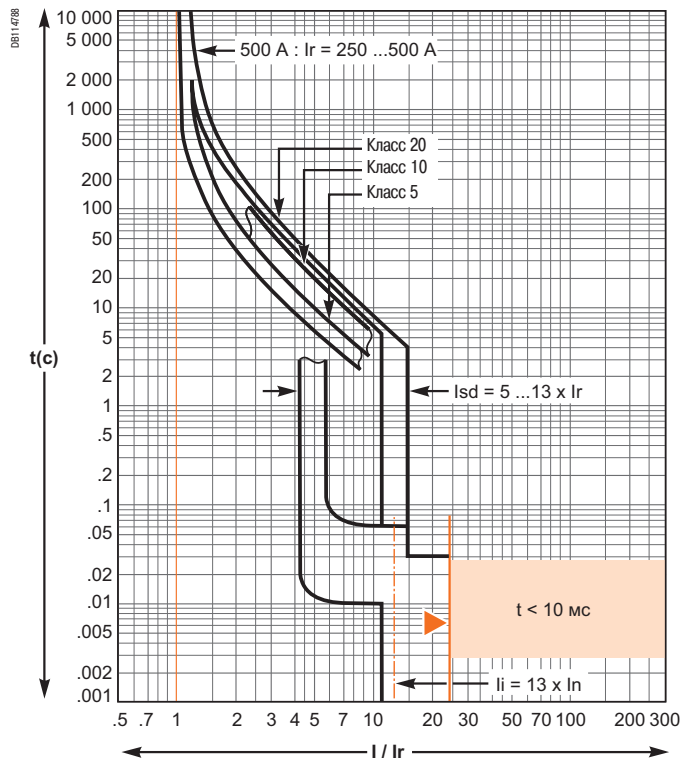
Micrologic 2.3 М - 500 А
