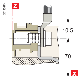
NSX100 - 250
