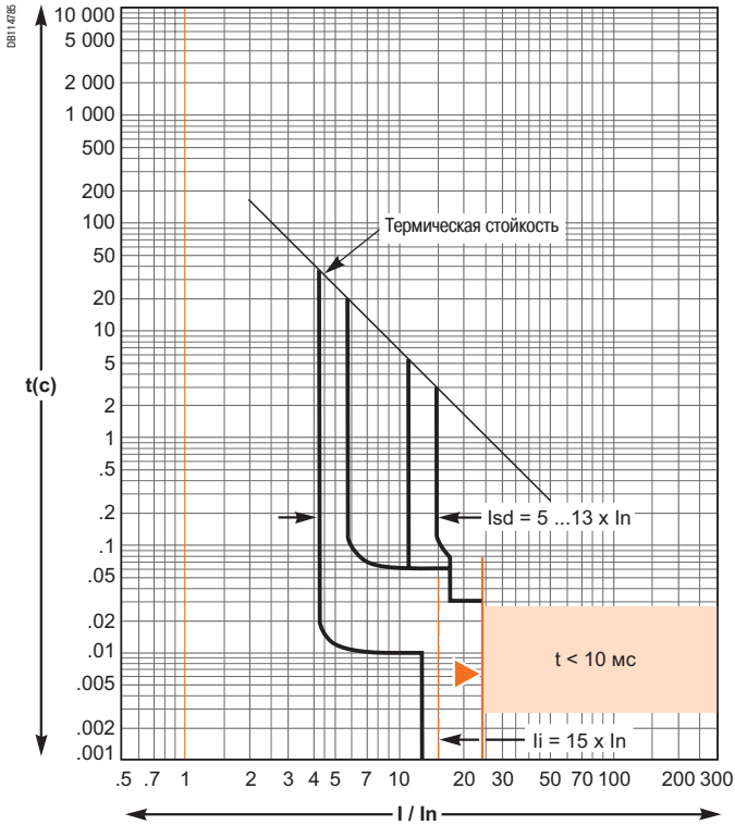
Micrologic 1.3 М - 320 А
