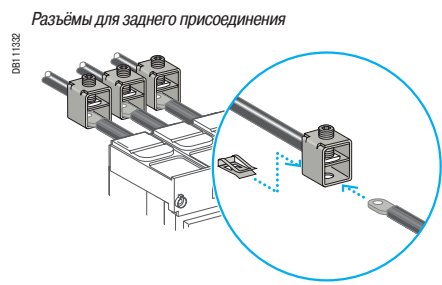
Присоединение кабелей без наконечников к NSX100 - 250
