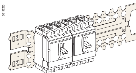
Крепление на монтажной плате Prisma
