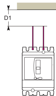
Аппараты с разделителями полюсов или длинной клеммной заглушкой
