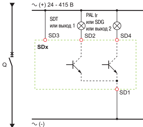
Электромонтажная схема модуля SDx
