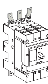
Переднее присоединение с расширителями полюсов
