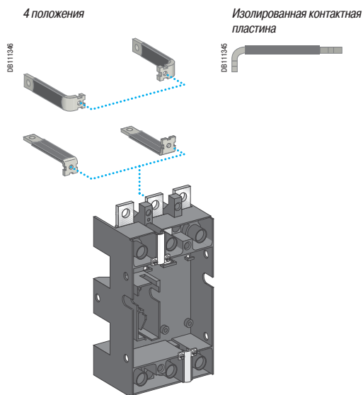
Переднее присоединение
