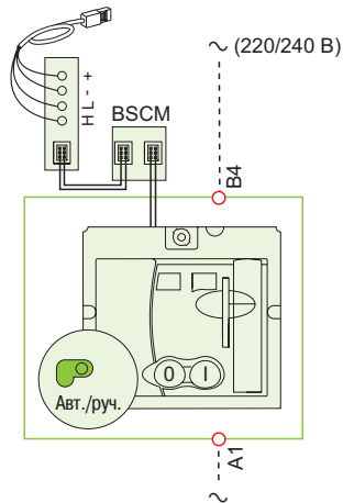
Коммутационный мотор-редуктор (МТс)
