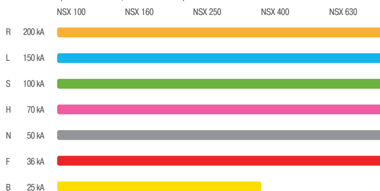
Уровни отключающей способности при 415 В
