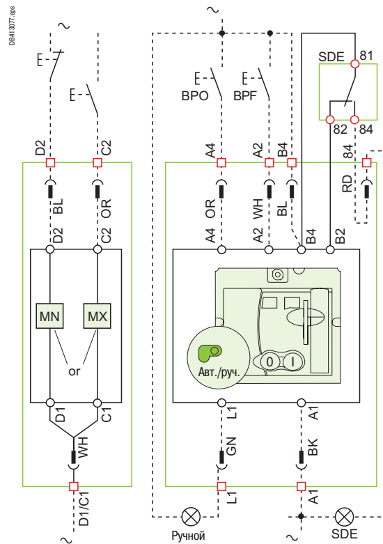
Мотор-редуктор (MT)
