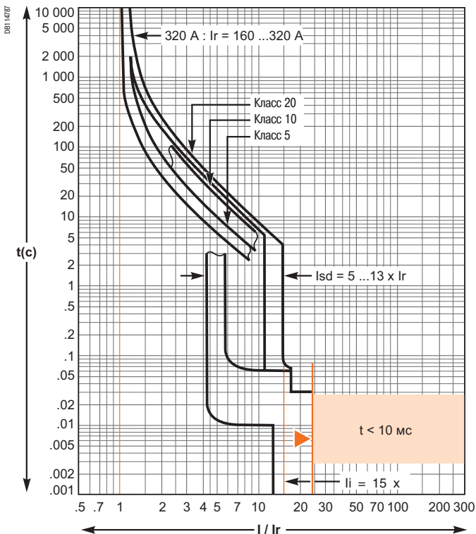
Micrologic 2.3 М - 320 А
