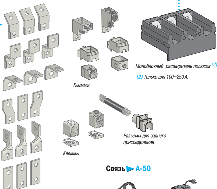
Дополнительные контактные пластины
