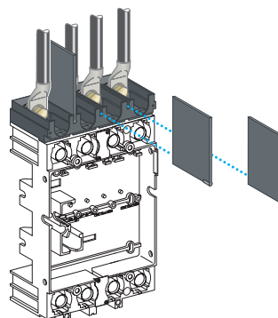
Переходник для цоколя 4-полюсного аппарата 400/630 A. Присоединение расширителей полюсов с разделителями полюсов
