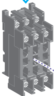
Блок втычных разъёмов, неподвижная часть
