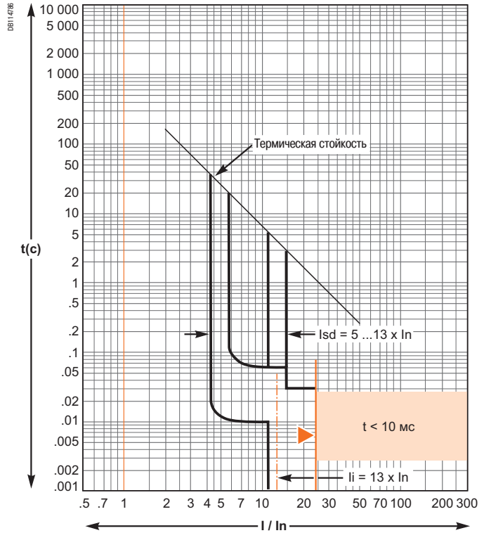
Micrologic 1.3 М - 500 А
