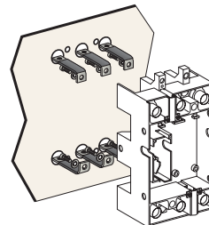
Заднее присоединение при креплении на задней панели (только с изолированной контактной пластиной)
